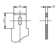
terminal F1
